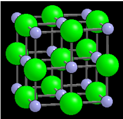
Kristallgitter des Salzes
